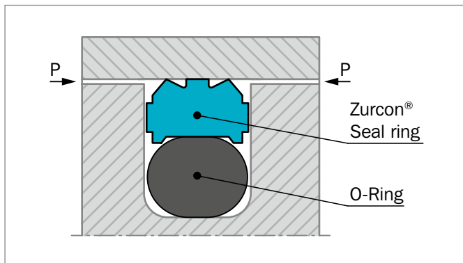
Figure 141: Zurcon® Wynseal
